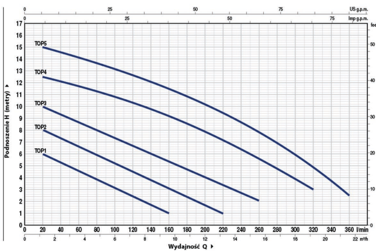
CHARAKTERYSTYKA POMP
